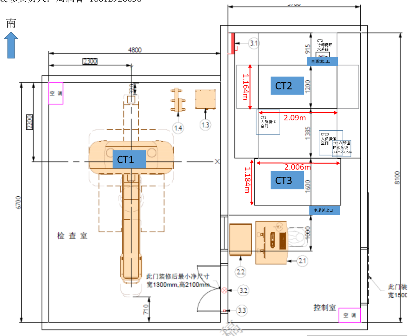
图一 房间布局设想
